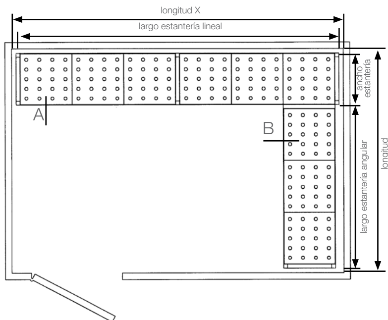
A-estantería lineal
